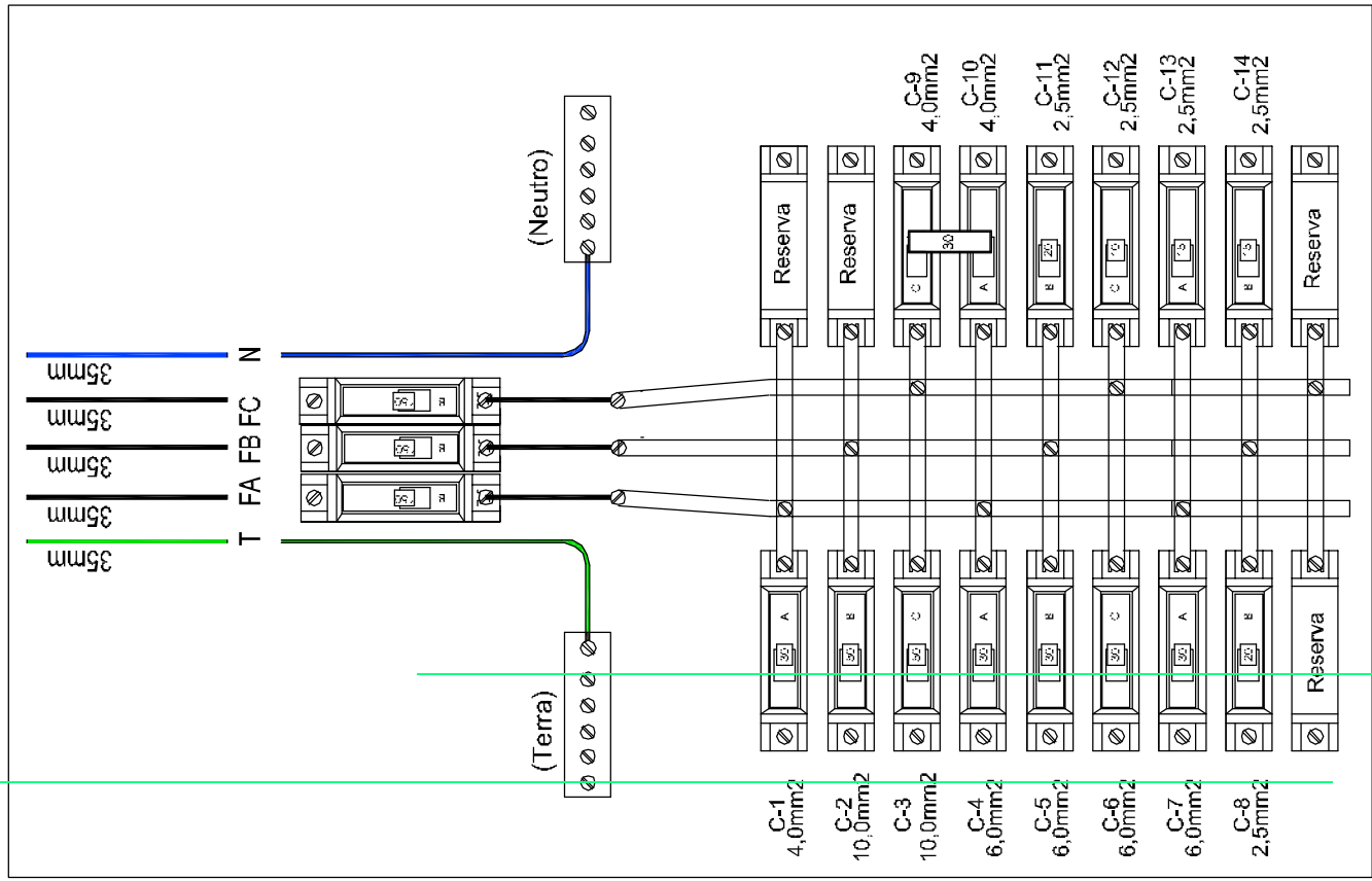
3 QUADRO DE DISTRIBUIÇÃO Sem escala
